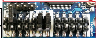
Bornier d'options
