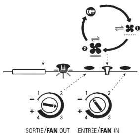
Détail des potentiomètres sur le VRC/VRE
